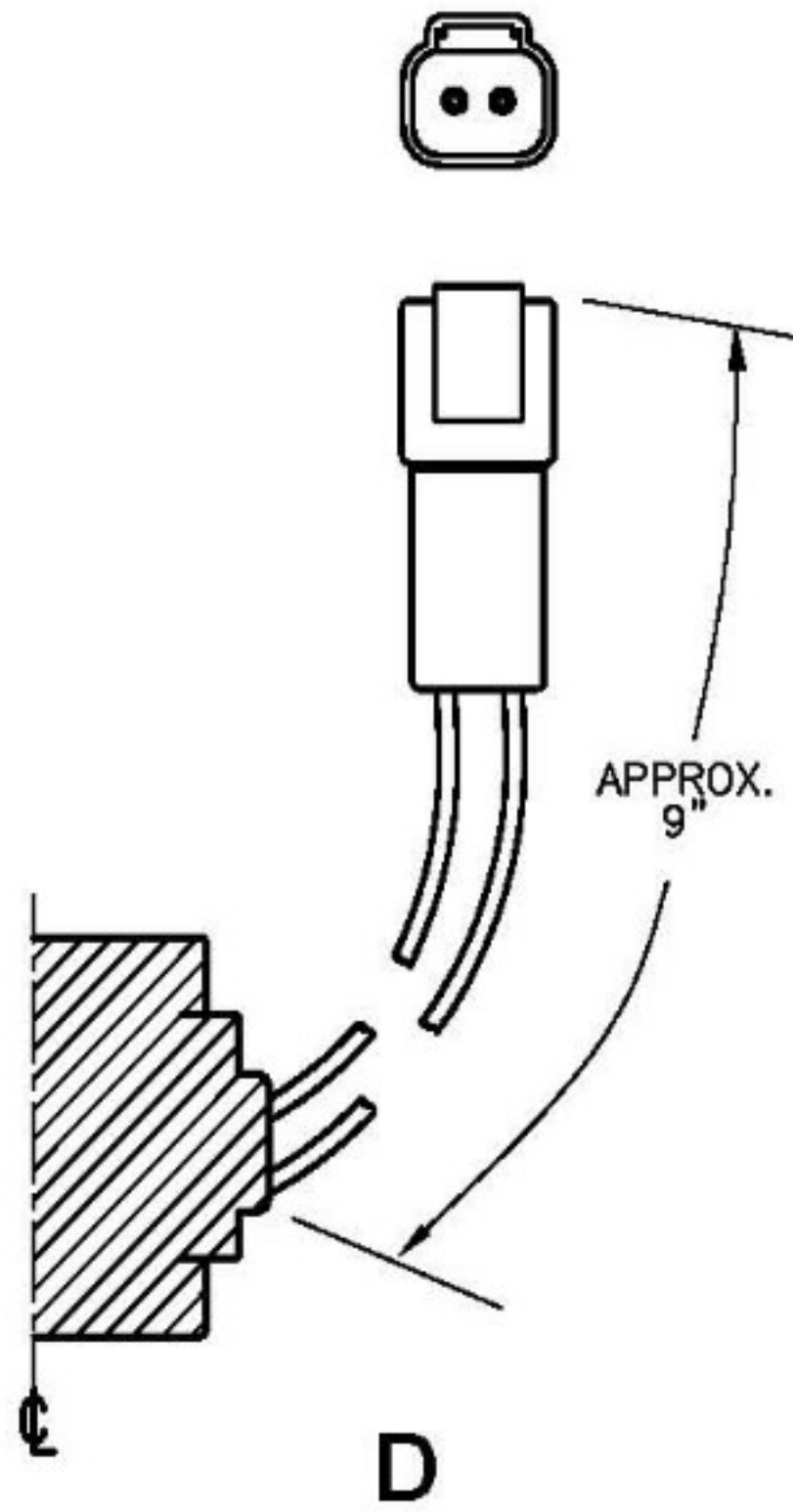
Deutsch DT04-2P Connector Mating Connector Deutsch - DT06-2S
